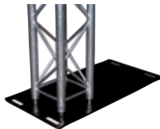
ASD embase lourde 80kg centrée ou décentrée pour H30V/X30D/H40V
